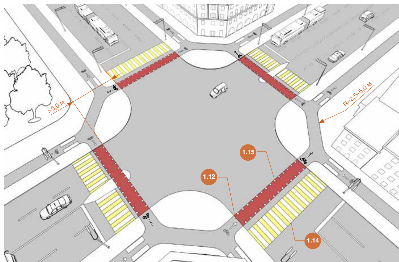
Рисунок 6.25 – Регулируемый перекресток. Улицы с односторонними велосипедными дорожками
