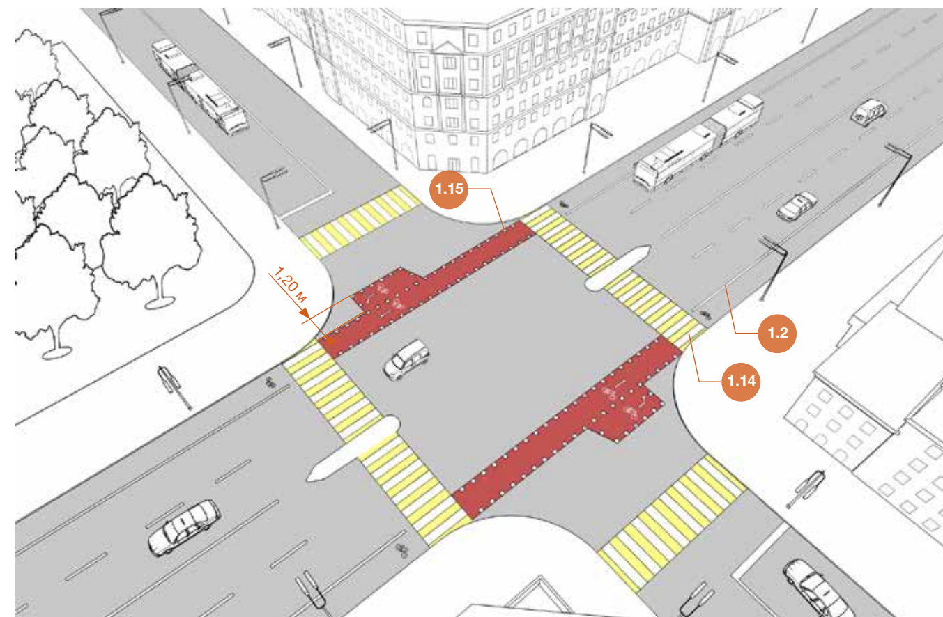
Рисунок 6.26 – Нерегулируемый перекресток. Главная дорога с велосипедной полосой
