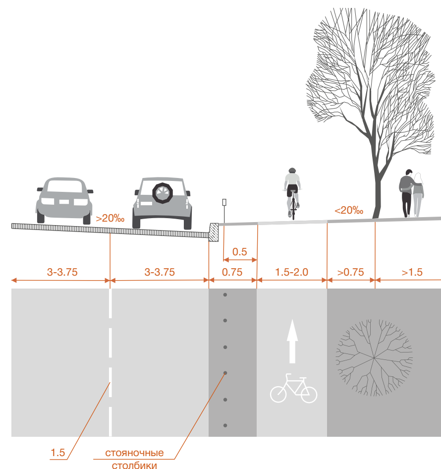
Рисунок 6.10 – Пример исполнения односторонней велосипедной дорожки с разделительной полосой и стояночными столбиками
