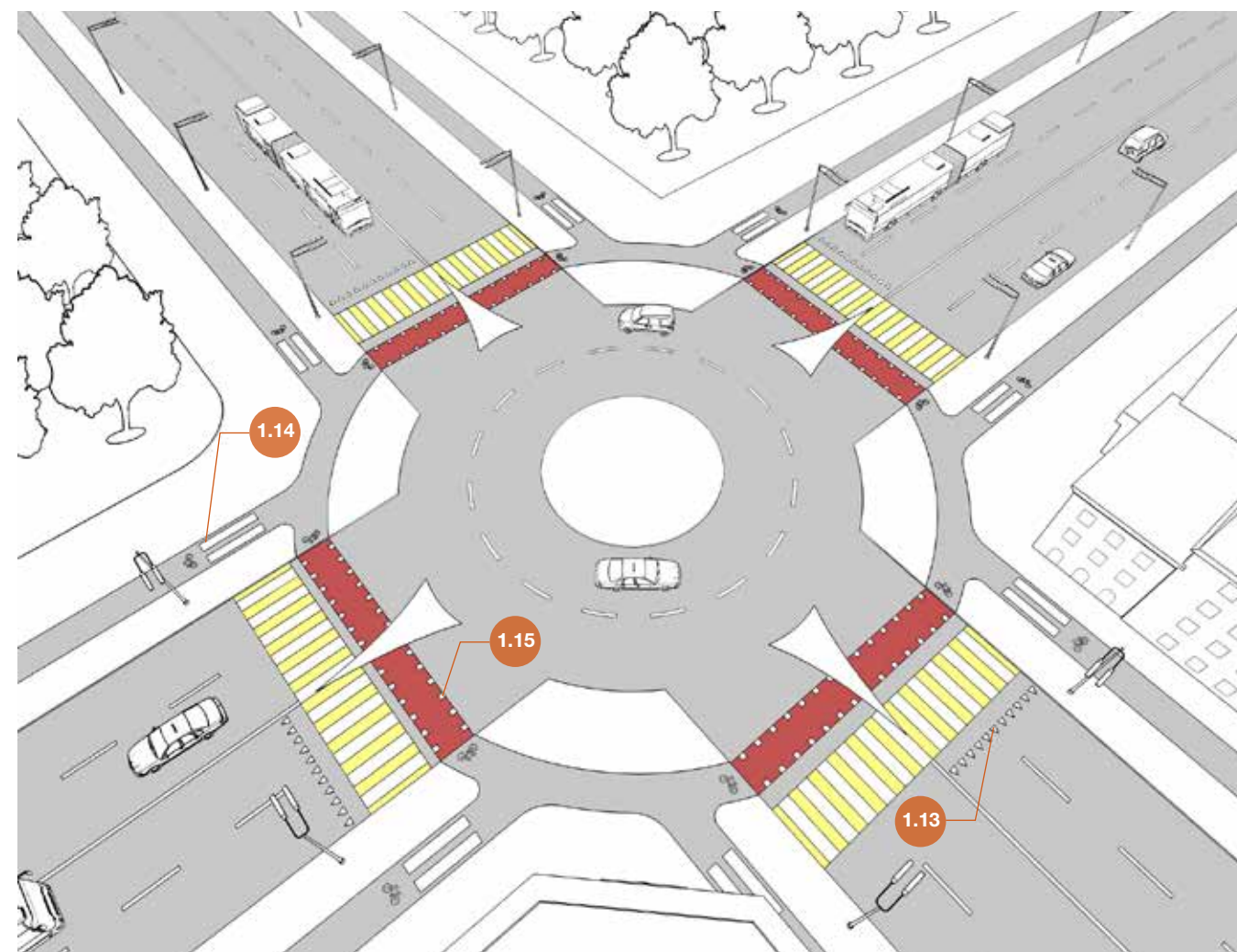
Рисунок 6.29 – Схема перекрестка с двухполосным круговым движением и приоритетом движения у транспорта, находящегося на круге
