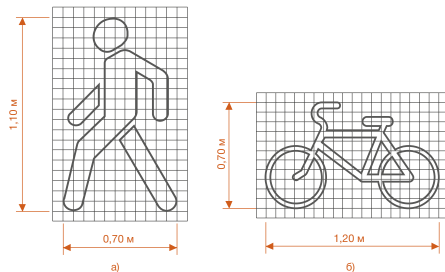
Рисунок 6.7 – Размеры разметки 1.23.2 и 1.23.3
