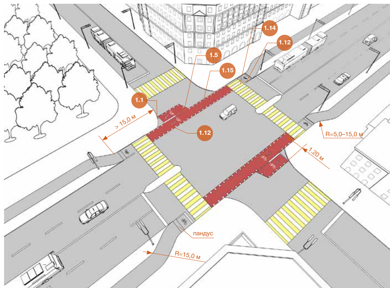
Рисунок 6.23 – Регулируемый перекресток. Главная дорога с велодорожкой, переходящей на перекрестке в велосипедную полосу
