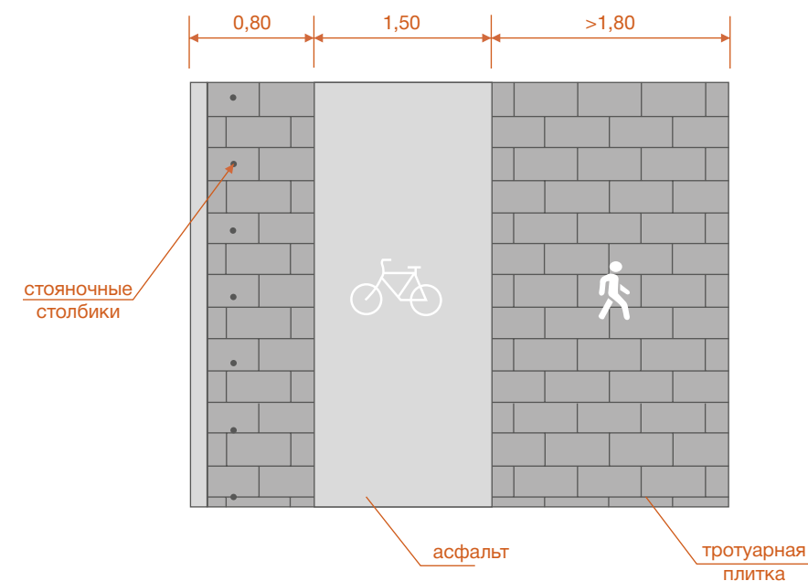
Рисунок 6.17 – Пример исполнения велосипедной дорожки из асфальтобетона
