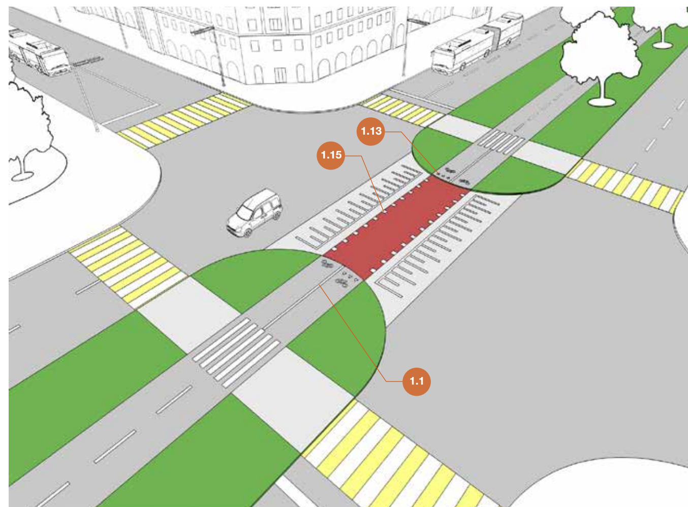
Рисунок 6.32 – Нерегулируемое пересечение с проездом через бульвар или разделительную полосу
