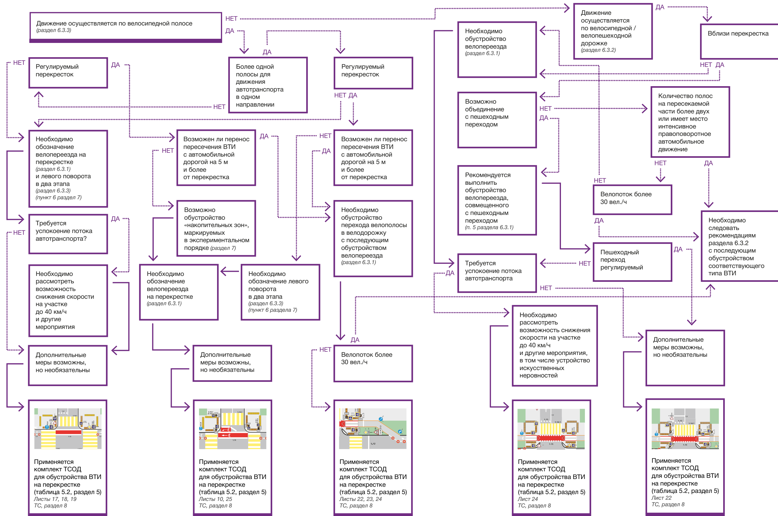
Схема 5.5 – Процесс организации ВТИ и выбора комплекса элементов обустройства на пересечениях с автомобильной дорогой при однонаправленном велопотоке от 16 до 50 вел./ч
