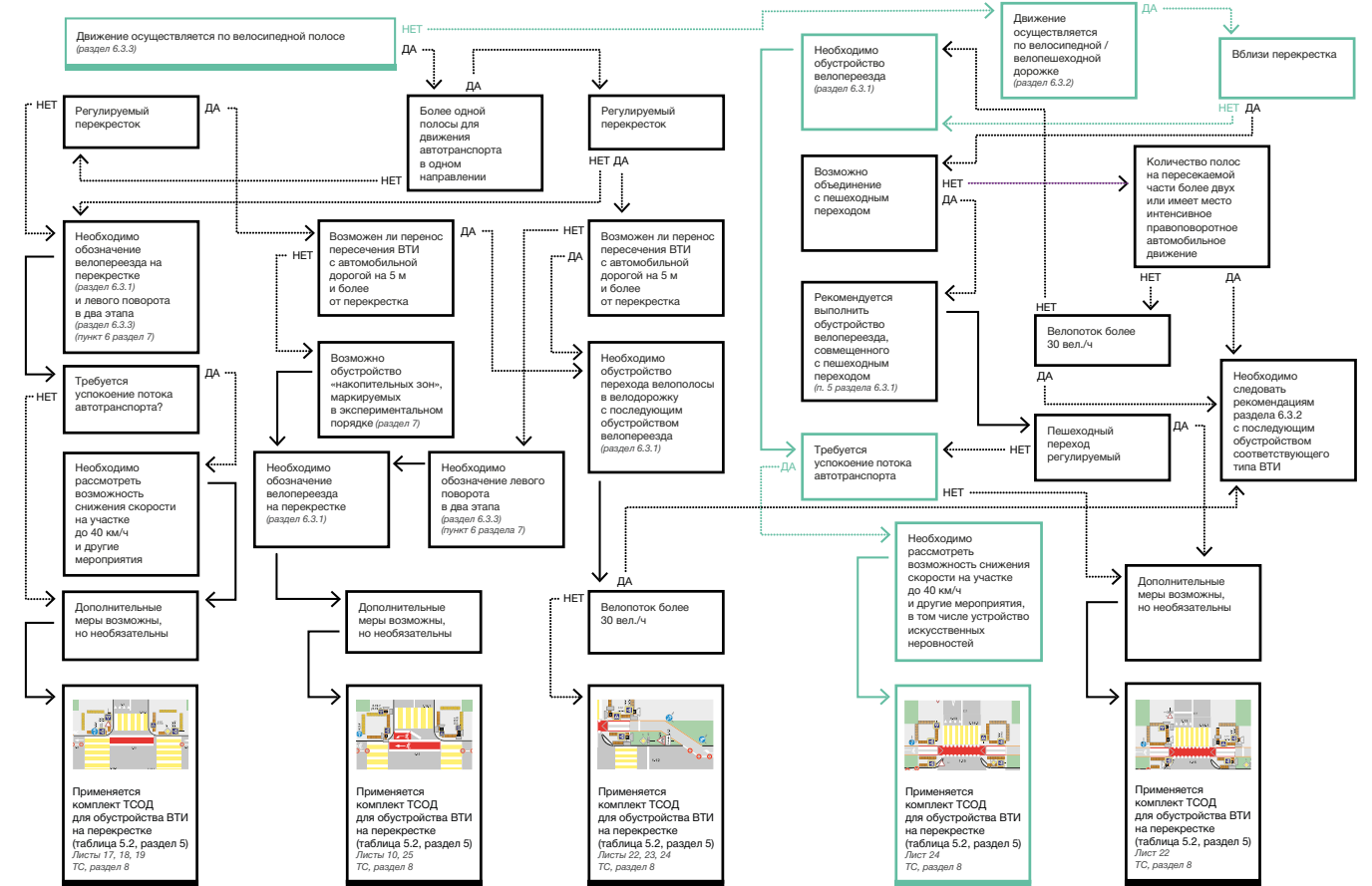
Рисунок 4.4 – Пример выбора варианта реализации ВТИ на пересечении
