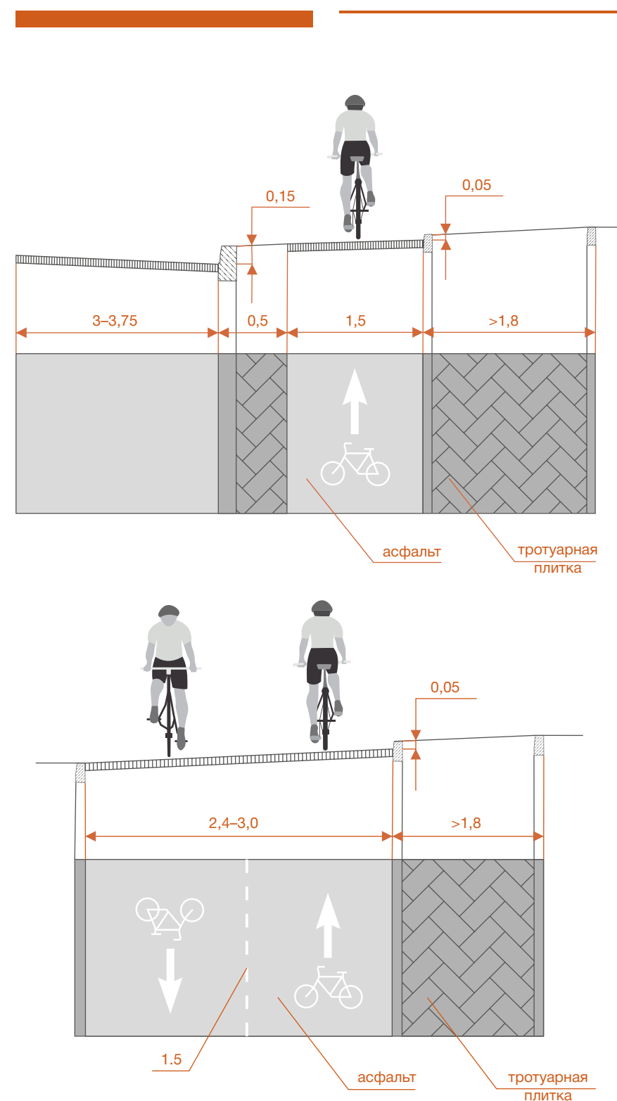
Рисунок 6.15 – Примеры устройства велосипедной дорожки, выполненной в разных уровнях по отношению к проезжей части и тротуару
