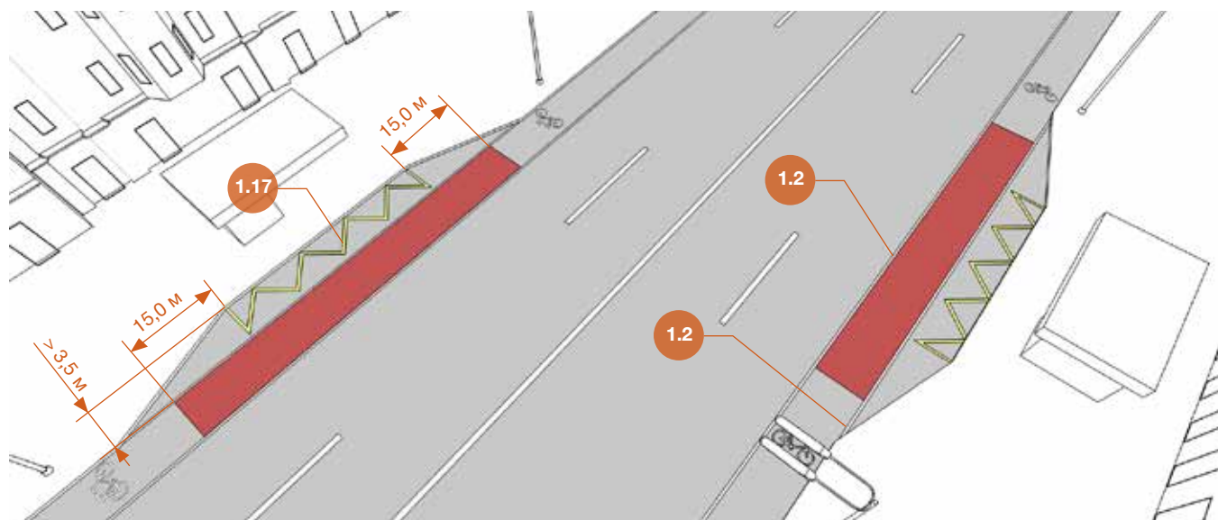
Рисунок 6.35 – Схемы размещения велосипедной полосы у остановки общественного транспорта
