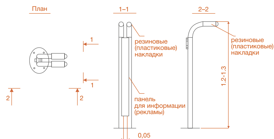
Рисунок 6.51 – Пример исполнения стойки технического осмотра велосипедов
