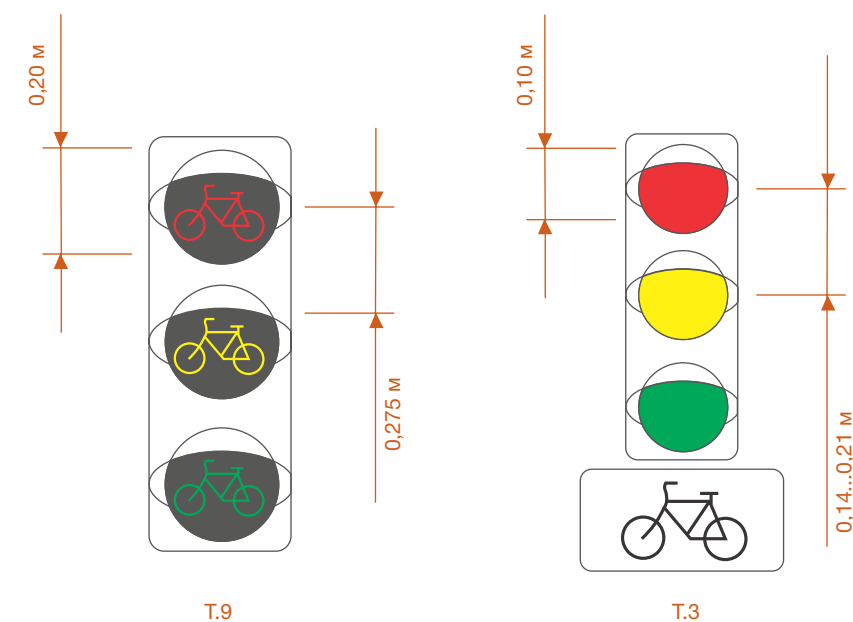
Рисунок 6.8 – Габариты светофоров Т.9 и Т.3 с табличкой 8.4.7
