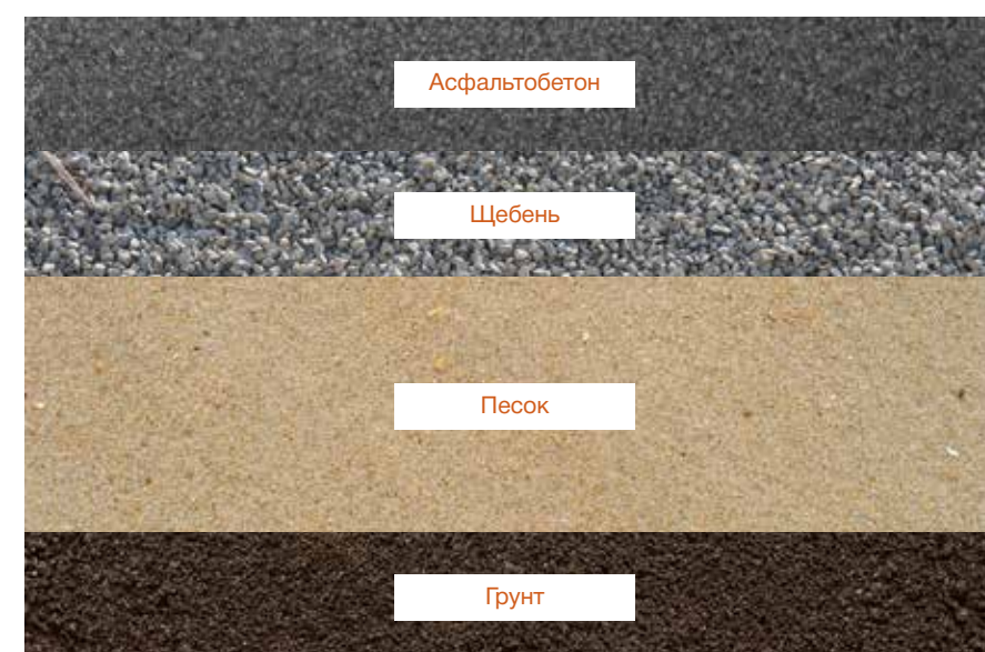
Рисунок 6.18 – Пример исполнения основания велосипедной дорожки
