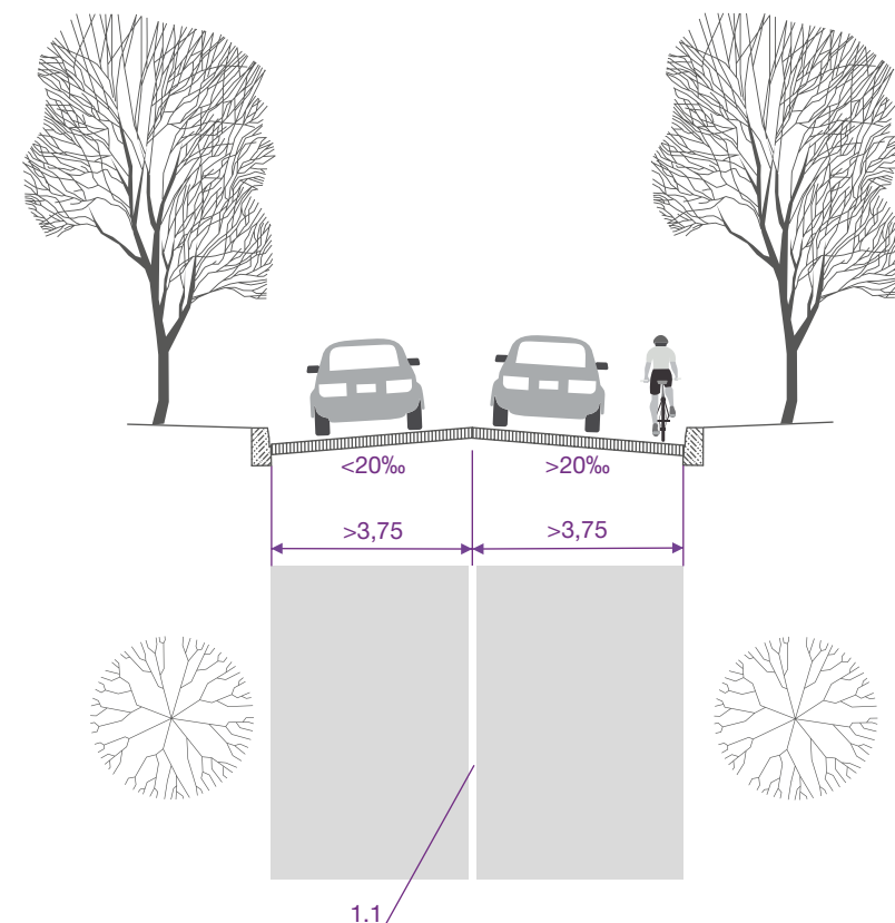
Рисунок 5.10 – Профиль улицы без выделенной ВТИ
