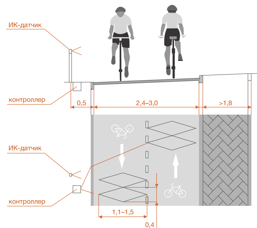
Рисунок 6.49 – Пример размещения комбинированного датчика двойной технологии – инфракрасной и индуктивной петли
