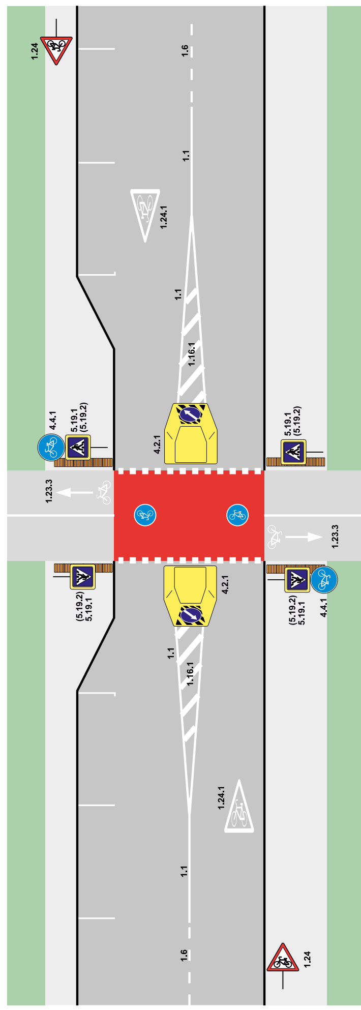
Лист 8 – Пересечение велосипедной дорожки (с двусторонним движением) с автомобильной дорогой
