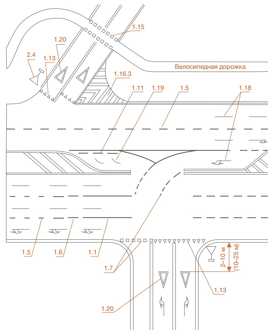
Рисунок 6.2 – Пример обозначения переезда для велосипедистов
