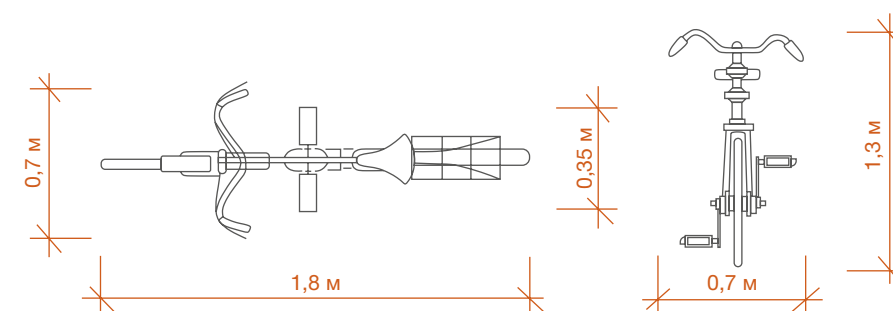
Рисунок 6.38 – Размеры стандартного велосипеда
