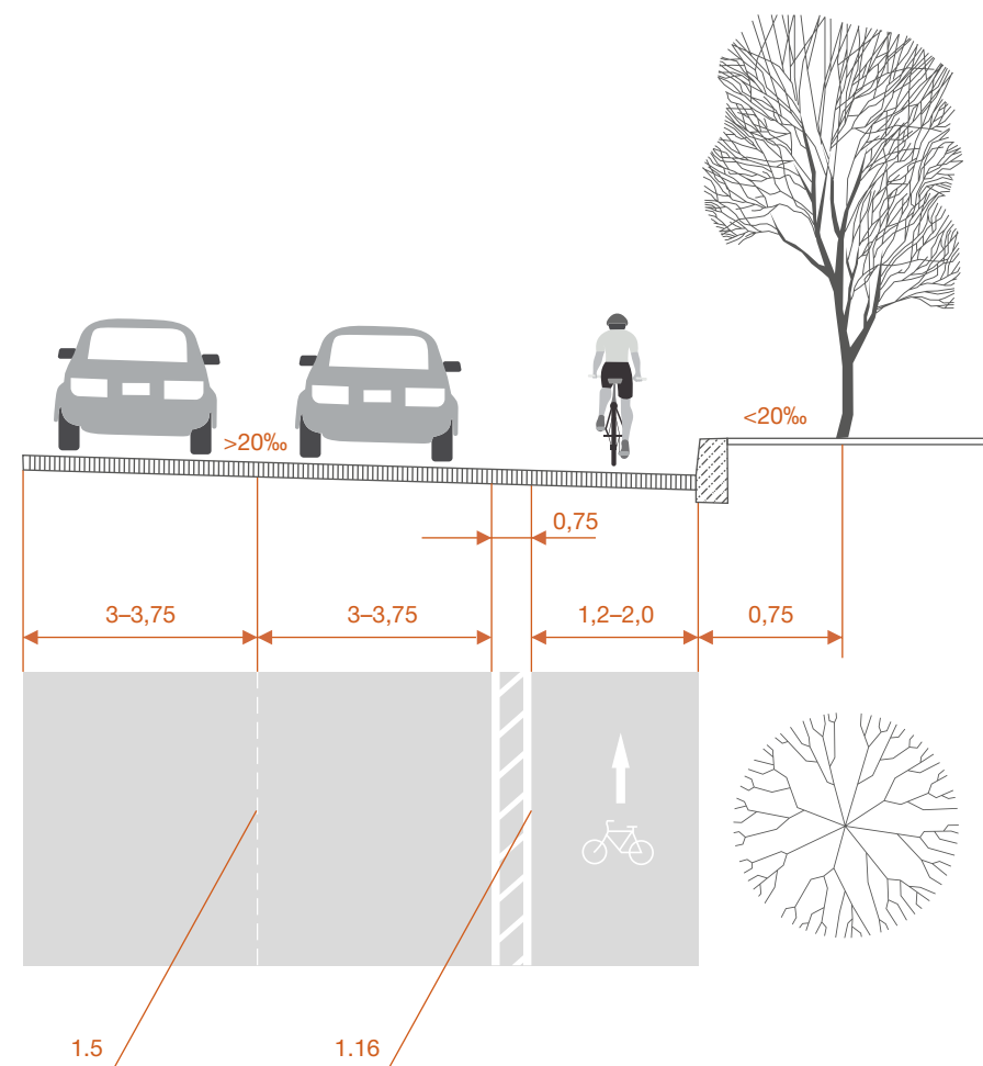
Рисунок 6.9 – Пример исполнения велосипедной полосы с нанесением «буферной зоны» для разделения велосипедных и транспортных потоков на улице с односторонним движением
