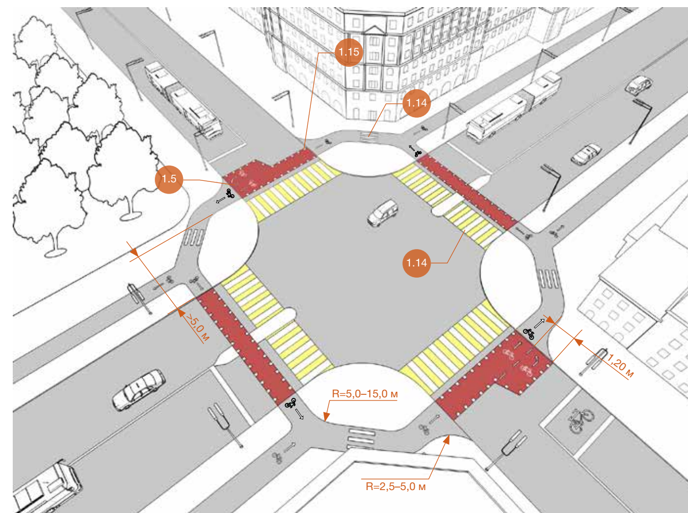
Рисунок 6.24 – Регулируемый перекресток. Главная дорога с велосипедной дорожкой с увеличением расстояния от оси главной дороги на перекрестке, второстепенная дорога с зоной для поворота в два действия
