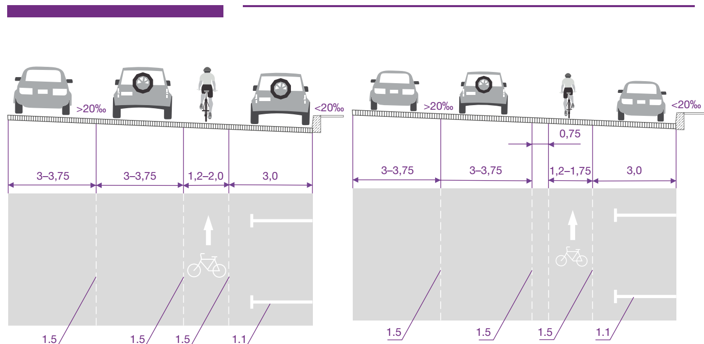
Рисунок 5.6 – Пример исполнения велосипедной полосы без «буферной зоны» (слева) и с «буферной зоной» (справа) вдоль парковочного кармана
