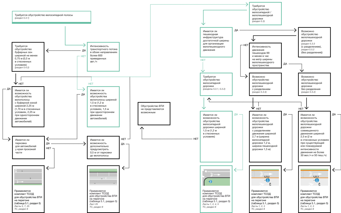
Рисунок 4.3 – Пример выбора варианта реализации ВТИ на перегоне
