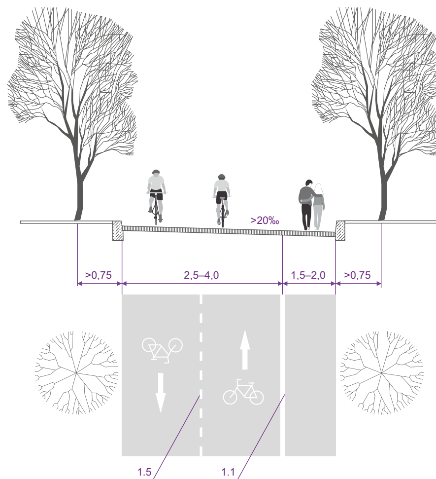
Рисунок 5.3 – Пример исполнения велопешеходной дорожки с разделением велосипедных и пешеходных потоков
