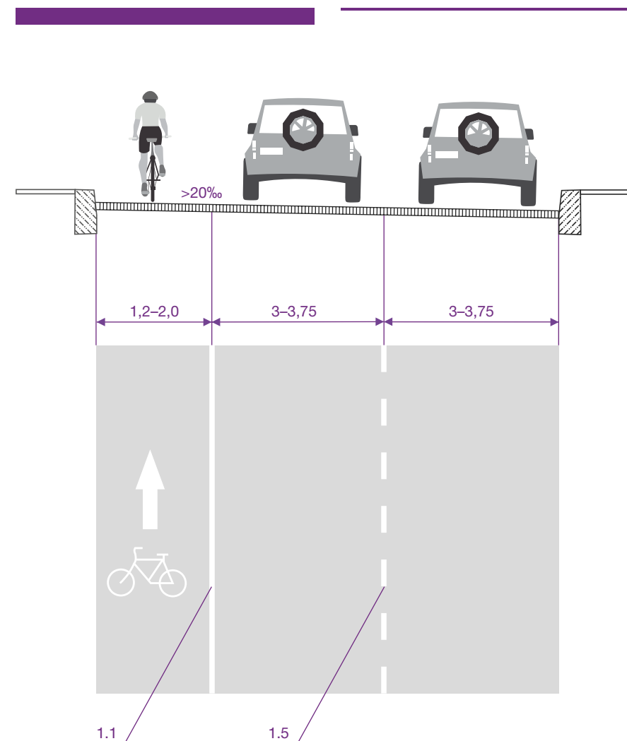
Рисунок 5.7 – Пример исполнения велосипедной полосы слева от проезжей части
