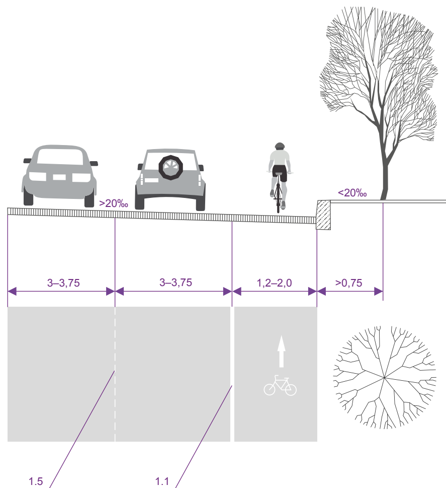
Рисунок 5.4 – Пример исполнения односторонней велосипедной полосы
