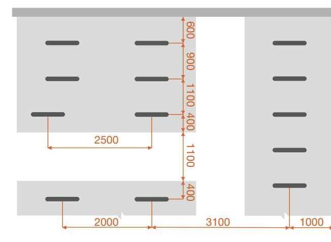
Рисунок 6.43 – Пример исполнения П-образных стоек велопарковки перпендикулярно боковым вертикальным конструкциям с обеспечением прохода велосипедистов
