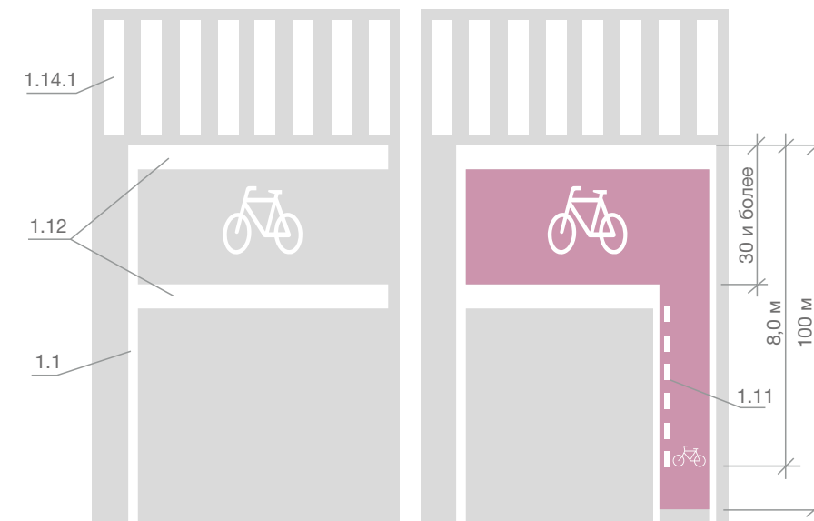
Рисунок 7.8 – Пример исполнения «накопительной зоны» перед перекрестком с помощью двух линий разметки 1.12 «стоп-линия», разметки 1.23.3 и нанесения цветного покрытия
