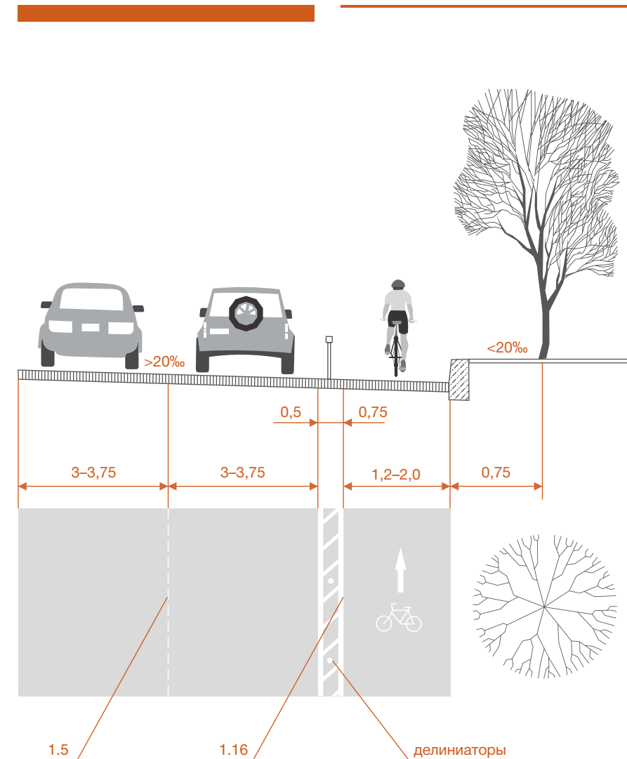
Рисунок 6.13 – Пример исполнения односторонней велосипедной дорожки с разделительной полосой и делиниаторами (столбиками)
