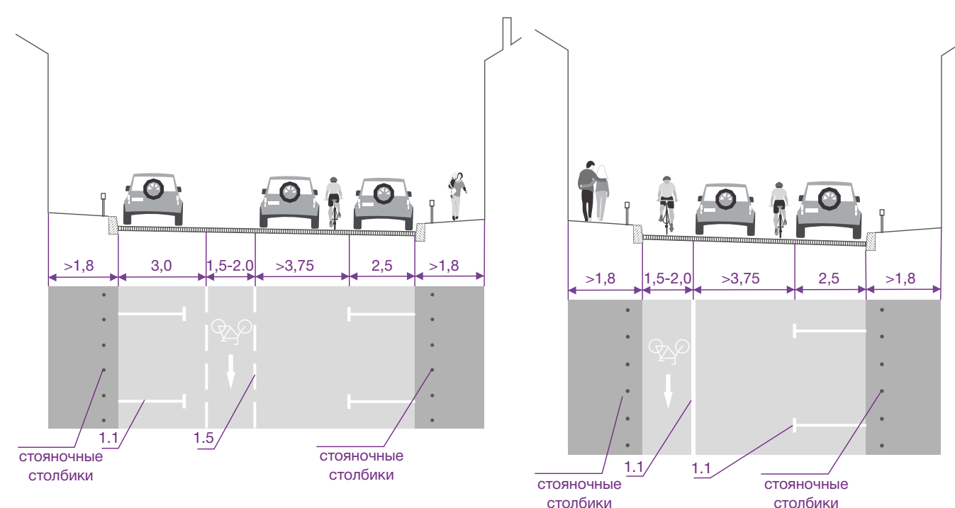
Пример исполнения велосипедной полосы встречного направления на улице с односторонним движением и карманами для паркинга с правой и левой стороны
