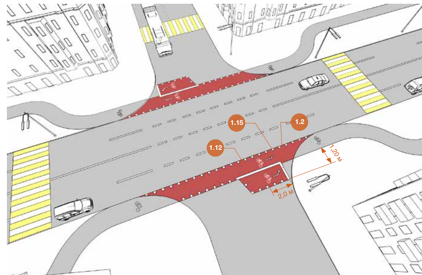
Рисунок 7.9 – Различные варианты исполнения устройства дополнительной полосы на перекрестке для осуществления велосипедистами левого поворота в два этапа
