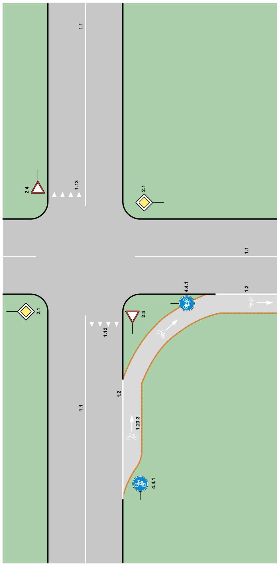
Лист 16 – Организация велосипедной дорожки непосредственно перед перекрестком с последующим поворотом направо
