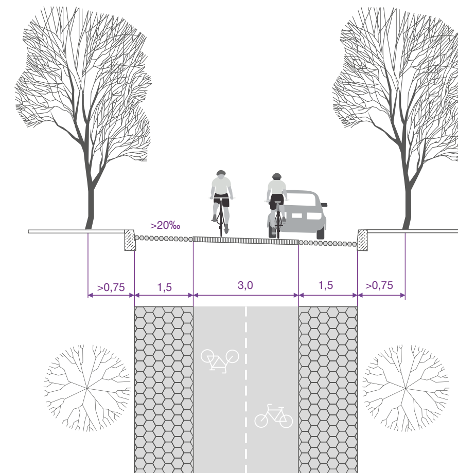
Рисунок 5.13 – Профиль велосипедной улицы с отличным типом покрытия
