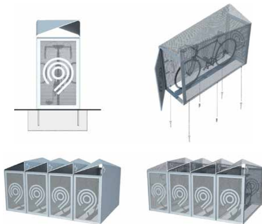
Рисунок 6.40 – Пример исполнения индивидуальной ячейки в г. Москве
