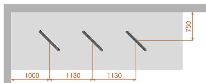
Рисунок 6.44 – Пример исполнения П-образных стоек велопарковки под углом 45 градусов к боковым вертикальным конструкциям
