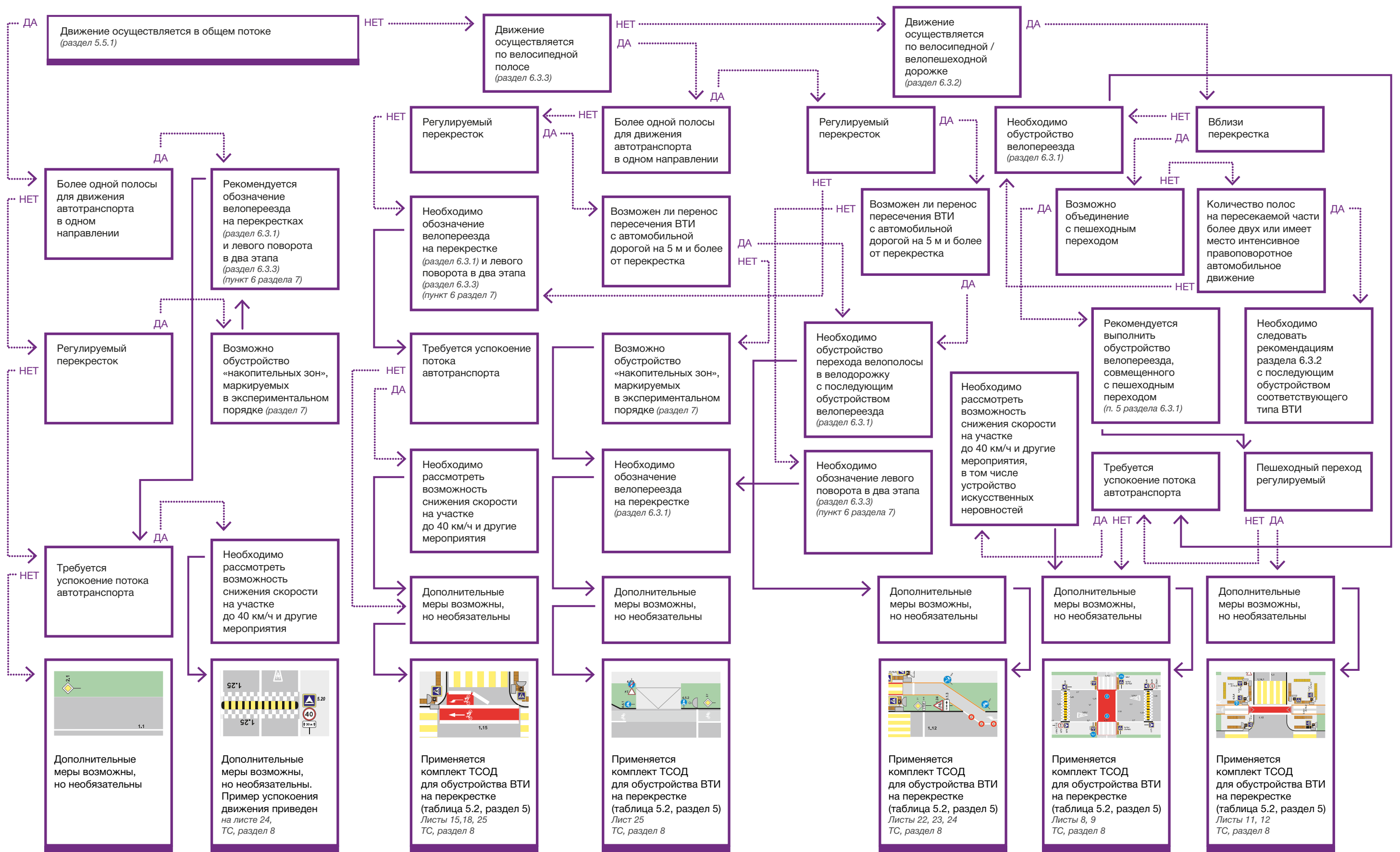
Схема 5.4 – Процесс организации ВТИ и выбора комплекса элементов обустройства на пересечениях с автомобильной дорогой при однонаправленном велопотоке до 15 вел./ч
