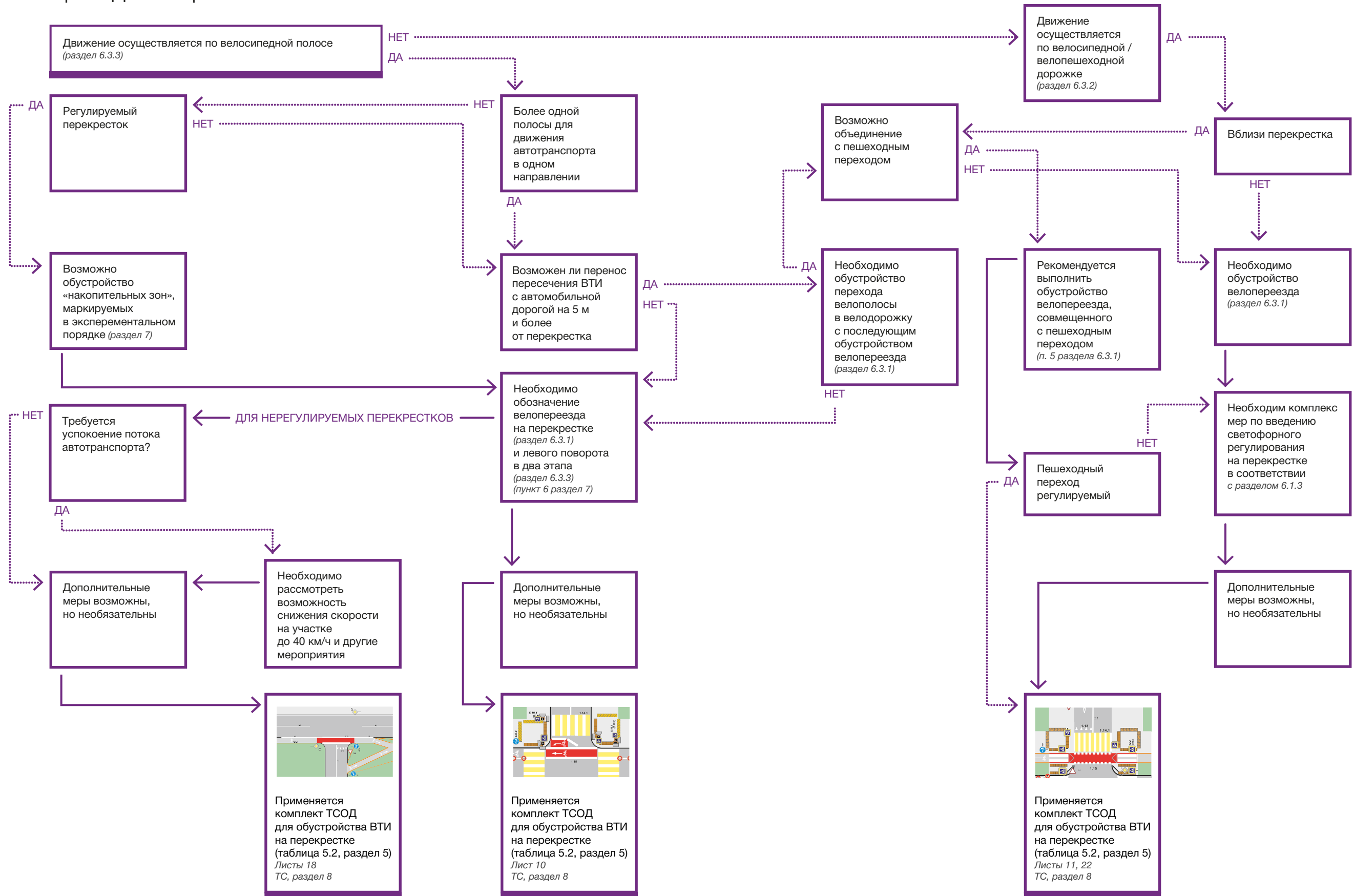
Схема 5.6 – Процесс организации ВТИ и выбора комплекса элементов обустройства на пересечениях с автомобильной дорогой при однонаправленном велопотоке более 51 вел./час
