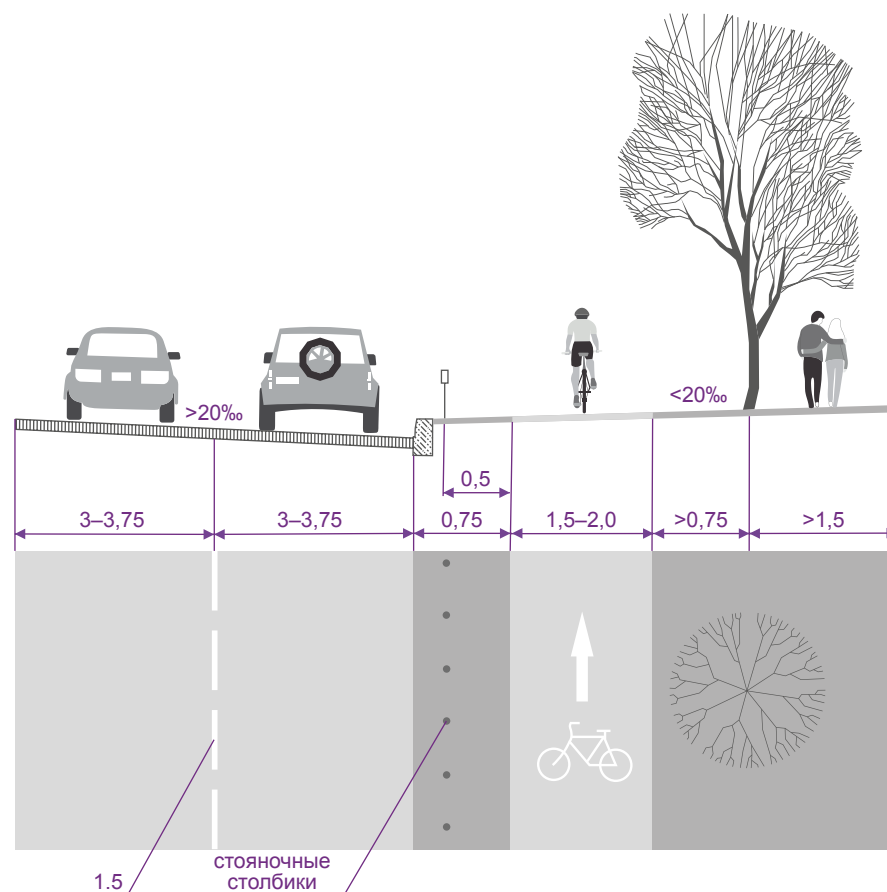
Рисунок 5.1 – Пример исполнения односторонней велосипедной дорожки
