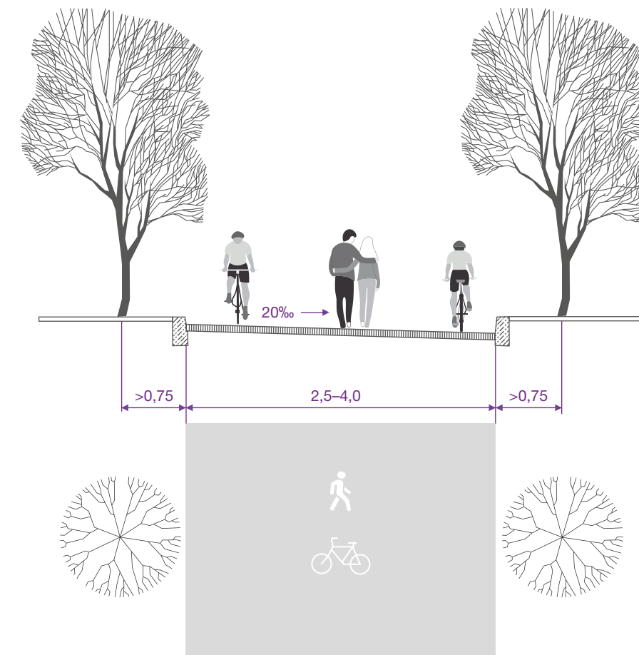
Рисунок 5.11 – Профиль велопешеходной дорожки без разделения велосипедных и пешеходных потоков
