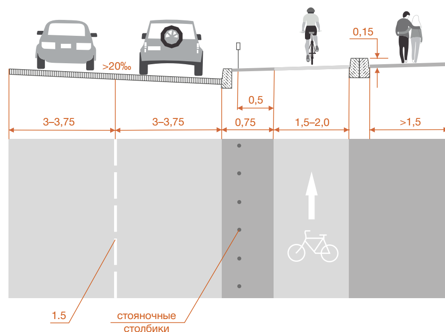
Рисунок 6.16 – Пример устройства велопешеходной дорожки с разделением
