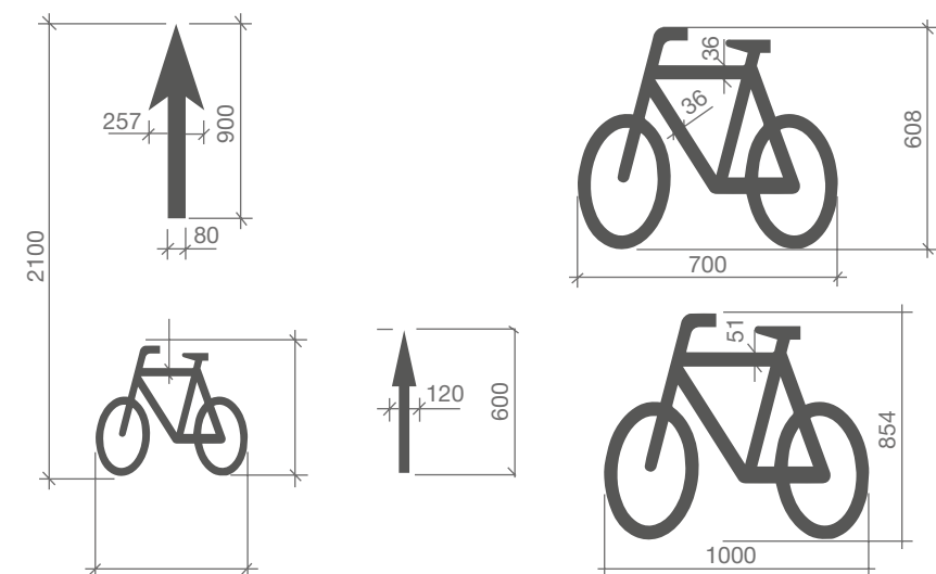
Рисунок 7.7 – Рекомендуемые размеры разметки 1.23.3 и 1.18 в экспериментальном порядке
