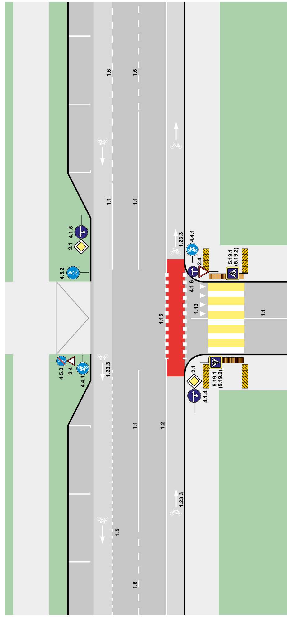
Лист 18 – Организация велосипедных полос с двух сторон от проезжей части с наличием парковки
