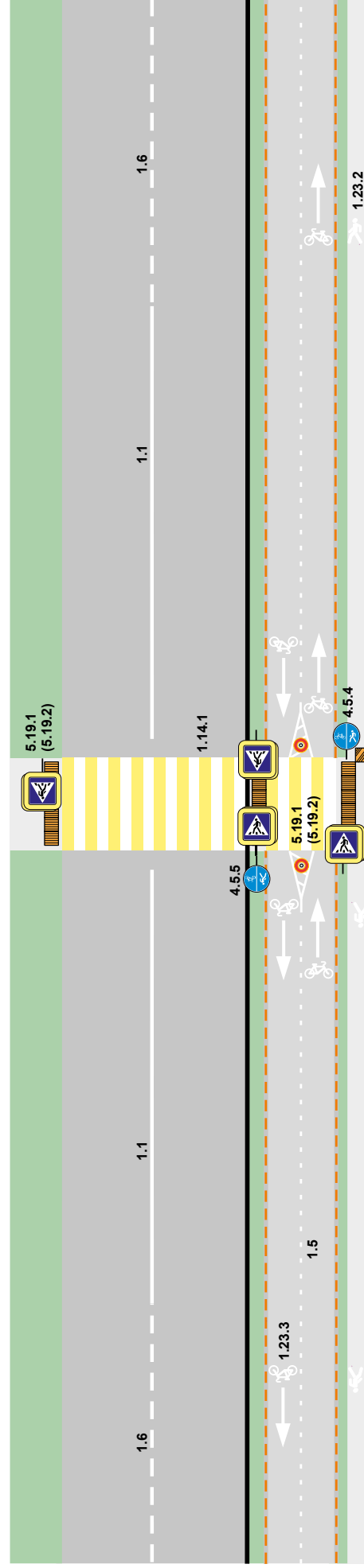
Лист 34 – Пересечение велодорожки с местом размещения пешеходного перехода
