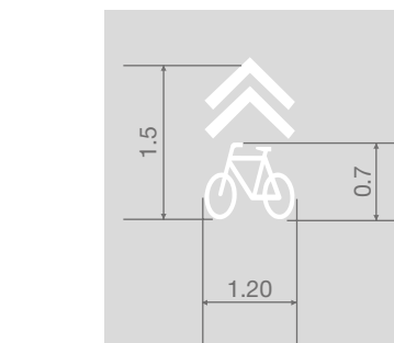
Рисунок 7.6 – Пример разметки для полосы общего пользования
