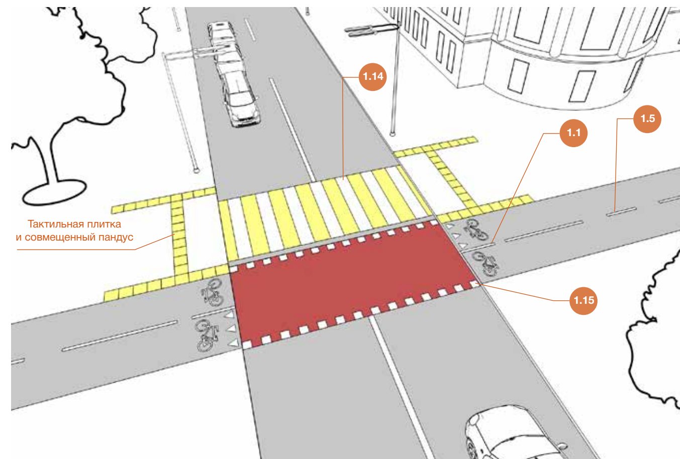
Рисунок 6.22 – Пример исполнения велосипедного переезда, совмещенного с пешеходным переходом
