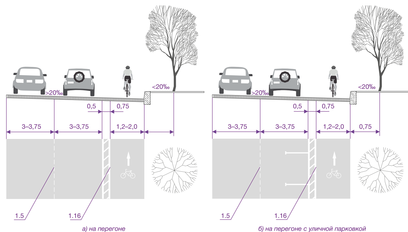
Рисунок 5.5 – Пример исполнения велосипедной полосы с буферной зоной
