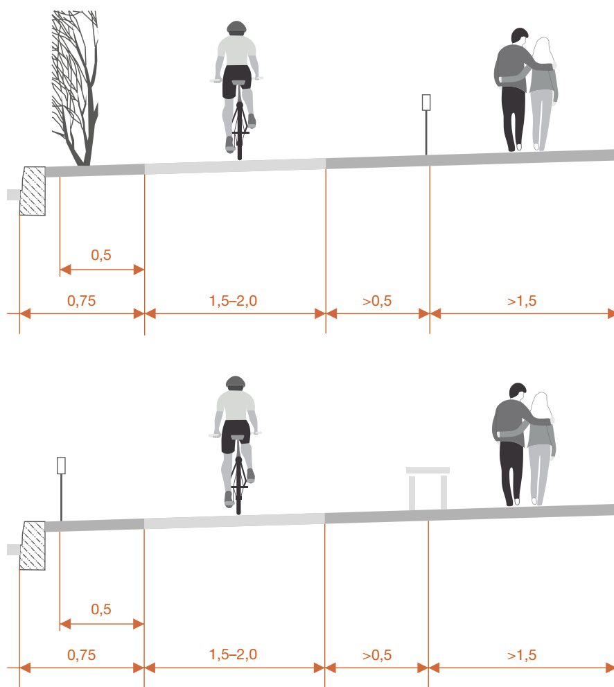
Рисунок 6.11 – Пример исполнения односторонней велосипедной дорожки с разделительной полосой и различными видами элементов
