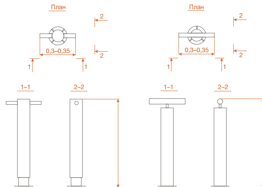
Рисунок 6.50 – Примеры станций ручной подкачки велосипедных шин
