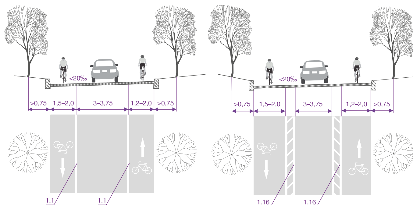
Пример исполнения велосипедных полос на улице с односторонним движением
