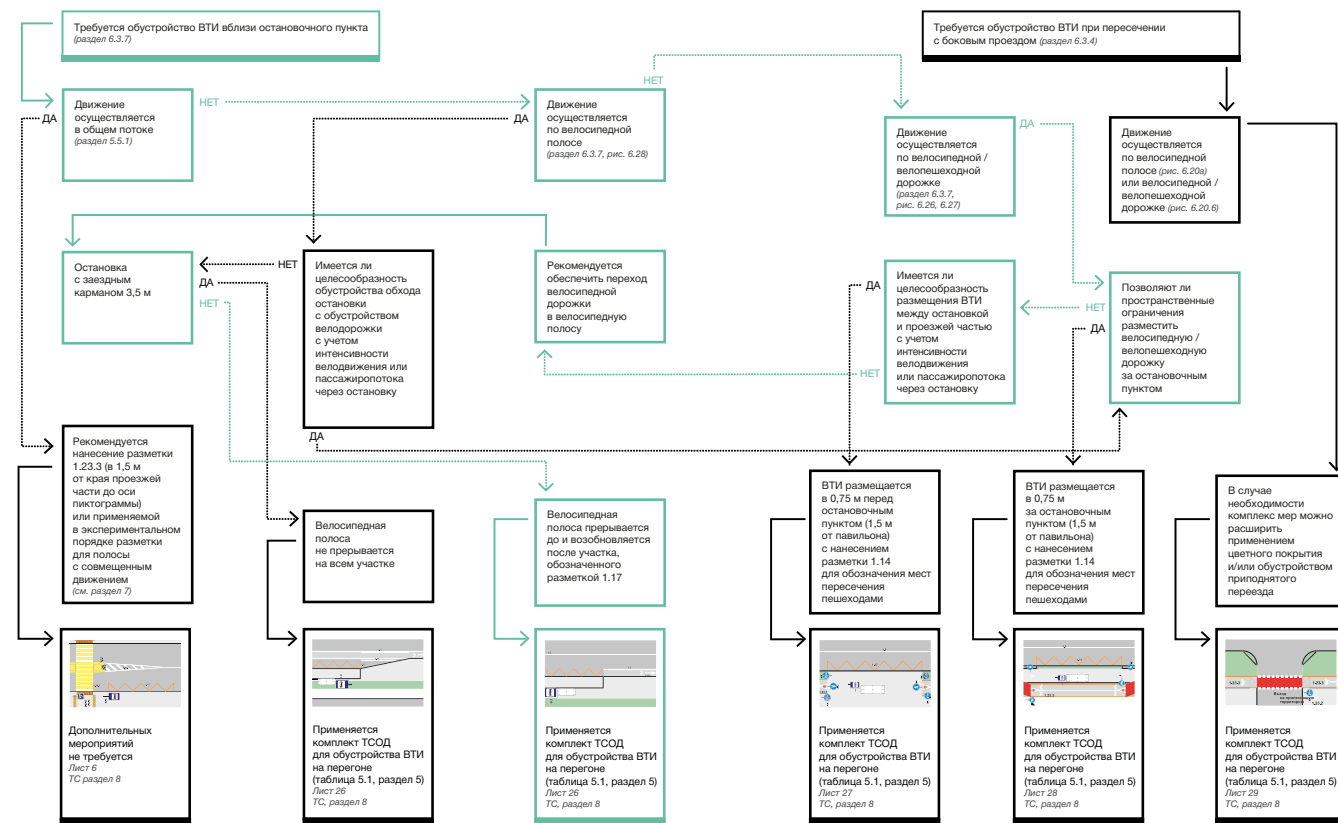
Рисунок 4.5 – Пример выбора варианта реализации ВТИ вблизи остановочного пункта городского пассажирского транспорта
