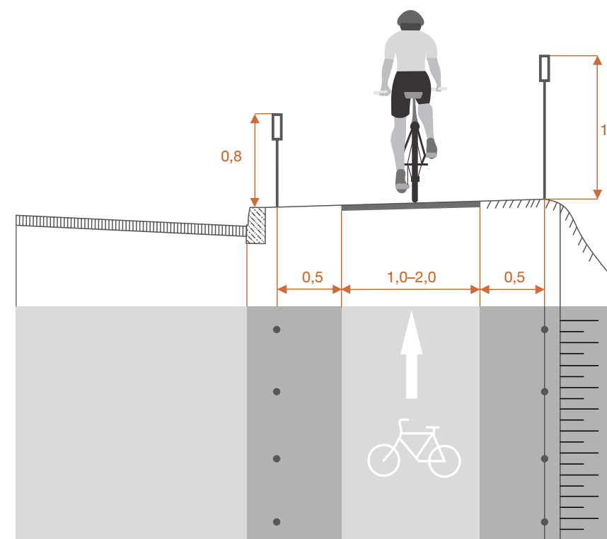
Рисунок 6.19 – Пример установки ограждения вдоль велосипедной дорожки
