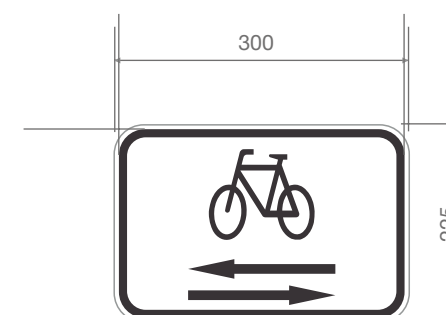
Рисунок 7.3 – Пример таблички, информирующей о направлении движения велосипедистов
