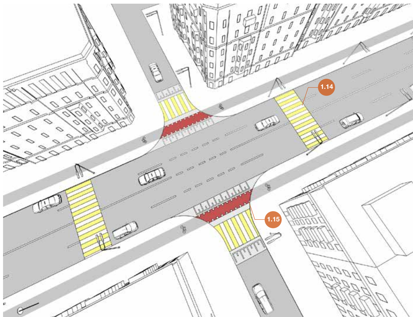
Рисунок 6.28 – Схема примыкания к улице с велосипедной дорожкой. Приподнятый велосипедный переезд, совмещенный с пешеходным переходом
