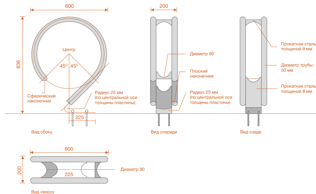
Рисунок 6.42 – Пример исполнения отдельно стоящей типовой рамы П-образной формы в г. Москве
