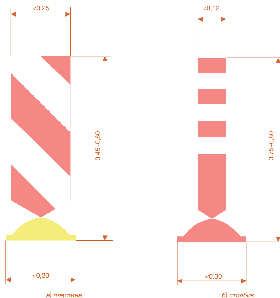
Рисунок 6.14 – Примеры исполнения делинаторов
