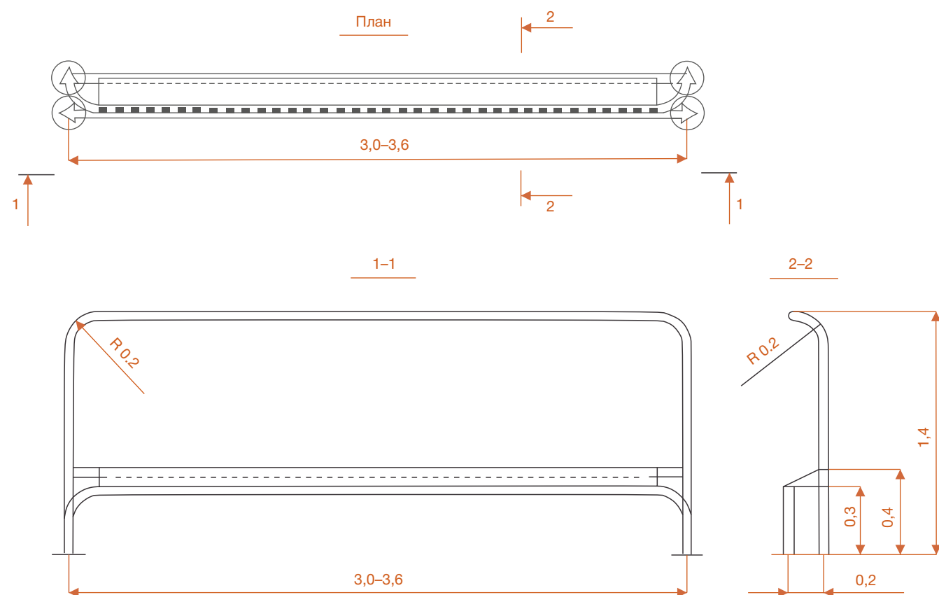
Рисунок 6.20 – Пример исполнения ограждений-держателей у перекрестков с регулируемым движением
