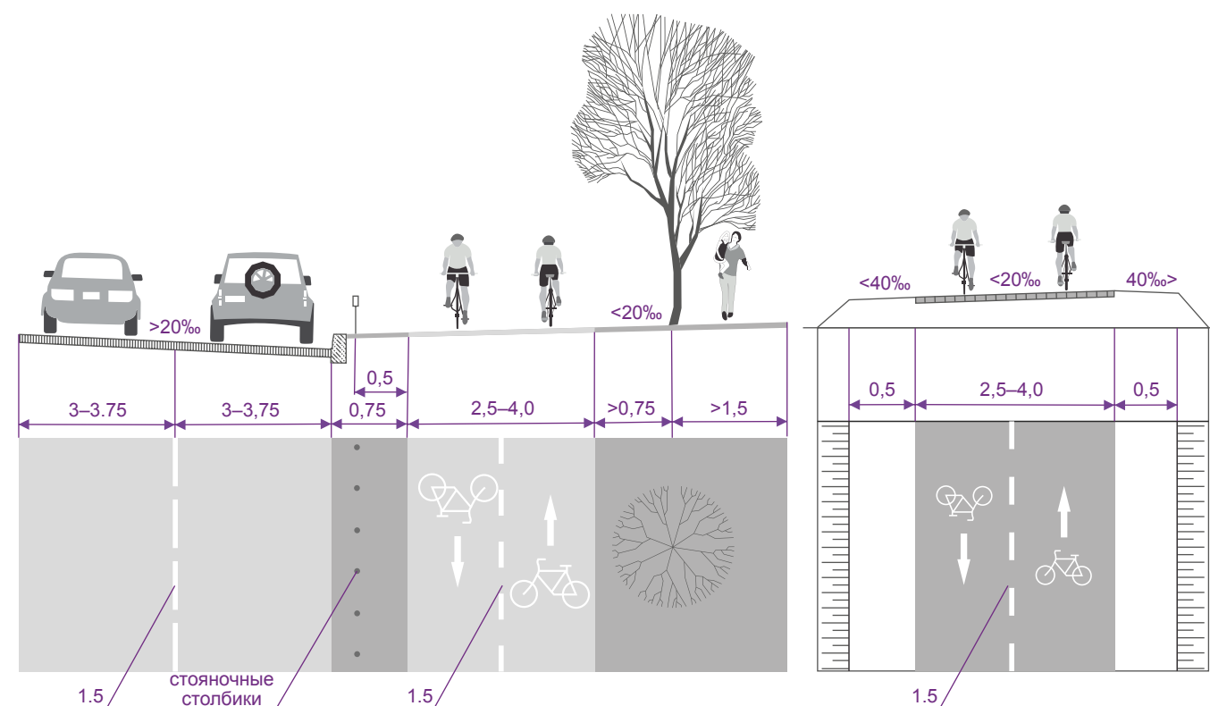
Рисунок 5.2 – Пример исполнения двухсторонней велосипедной дорожки с одной стороны проезжей части (слева) и на отдельном земляном полотне (справа)
